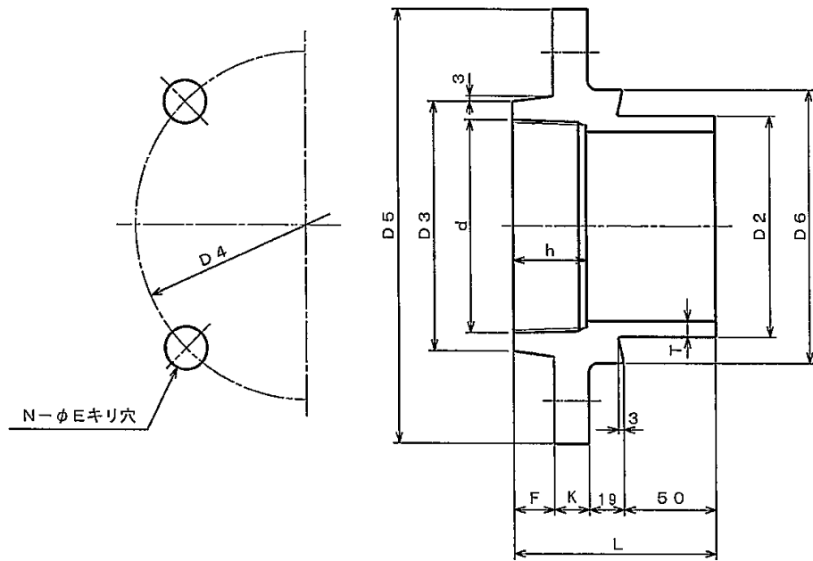
1形 寸法表
